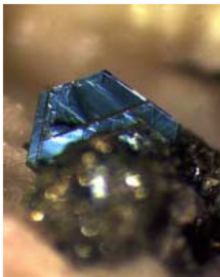
Polibasita sobre Cuarzo, Mina de Imiter, Morocco Fotografía de Gilles Levesse
